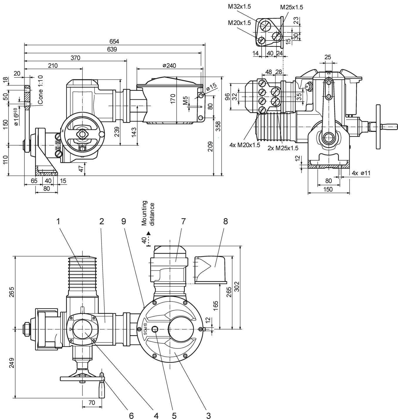
外形尺寸图
