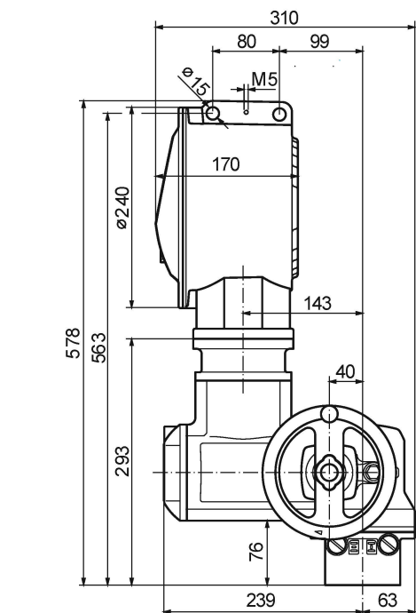
外形尺寸图
