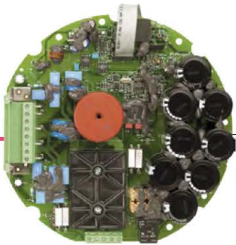
电源板
