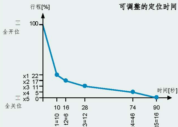
输出转速控制的实例
