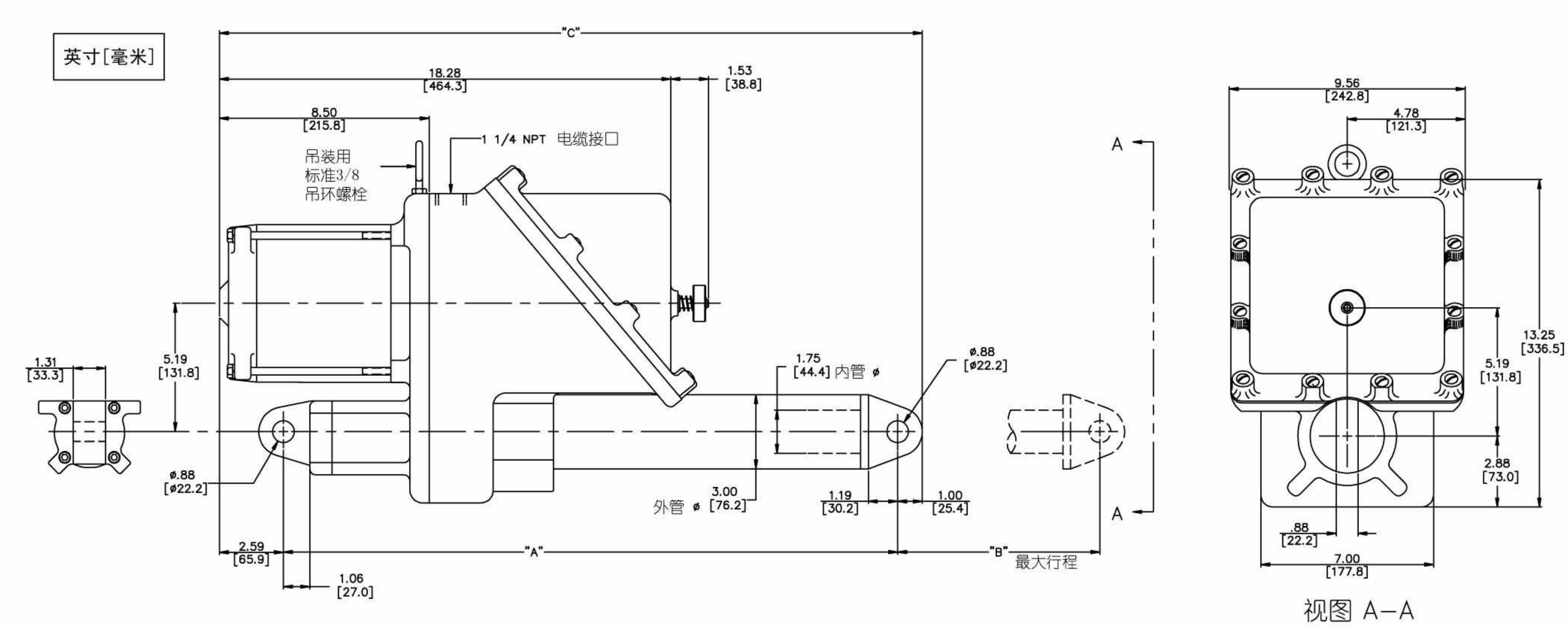
LA-2500 尺寸图
