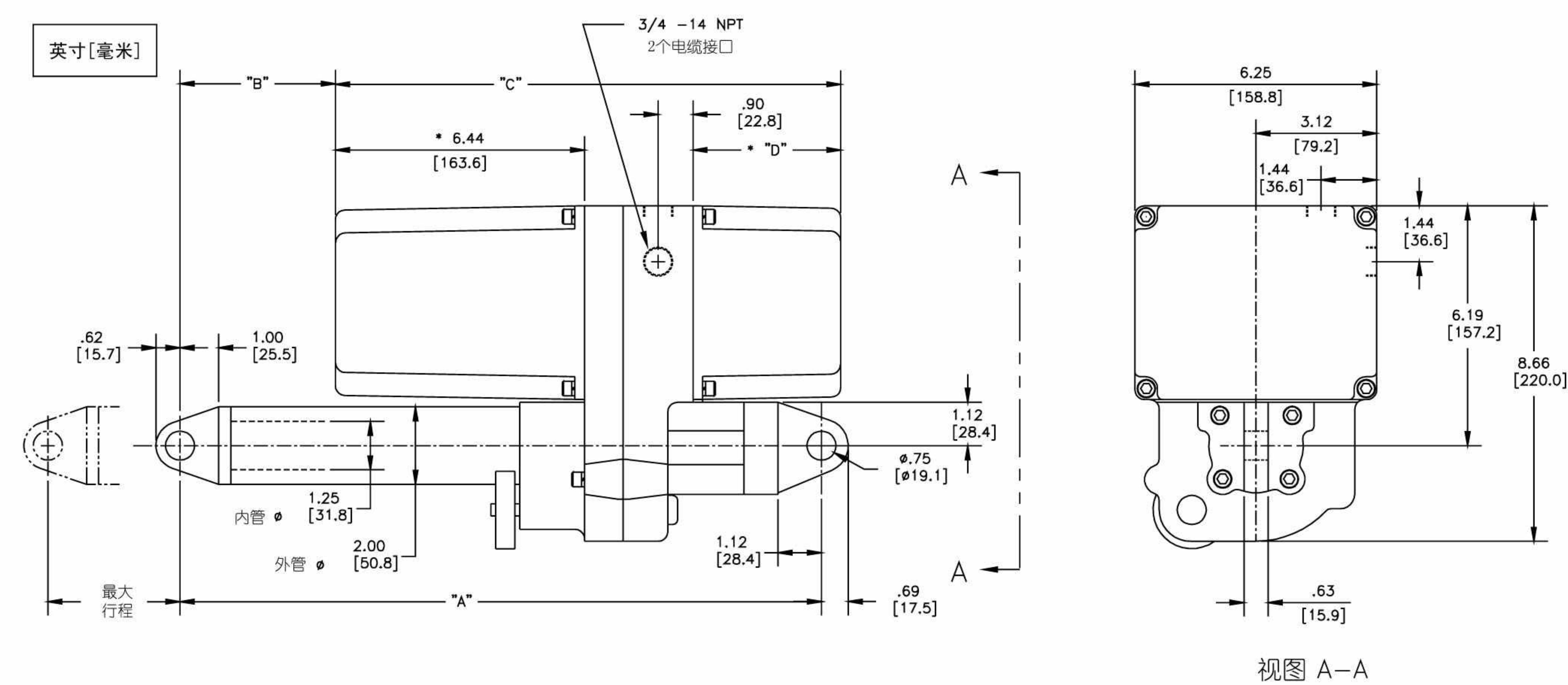
LA-2400 尺寸图
