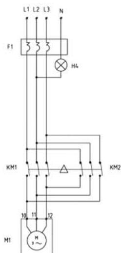
MOTOR POWER SUPPLY 马达电源
