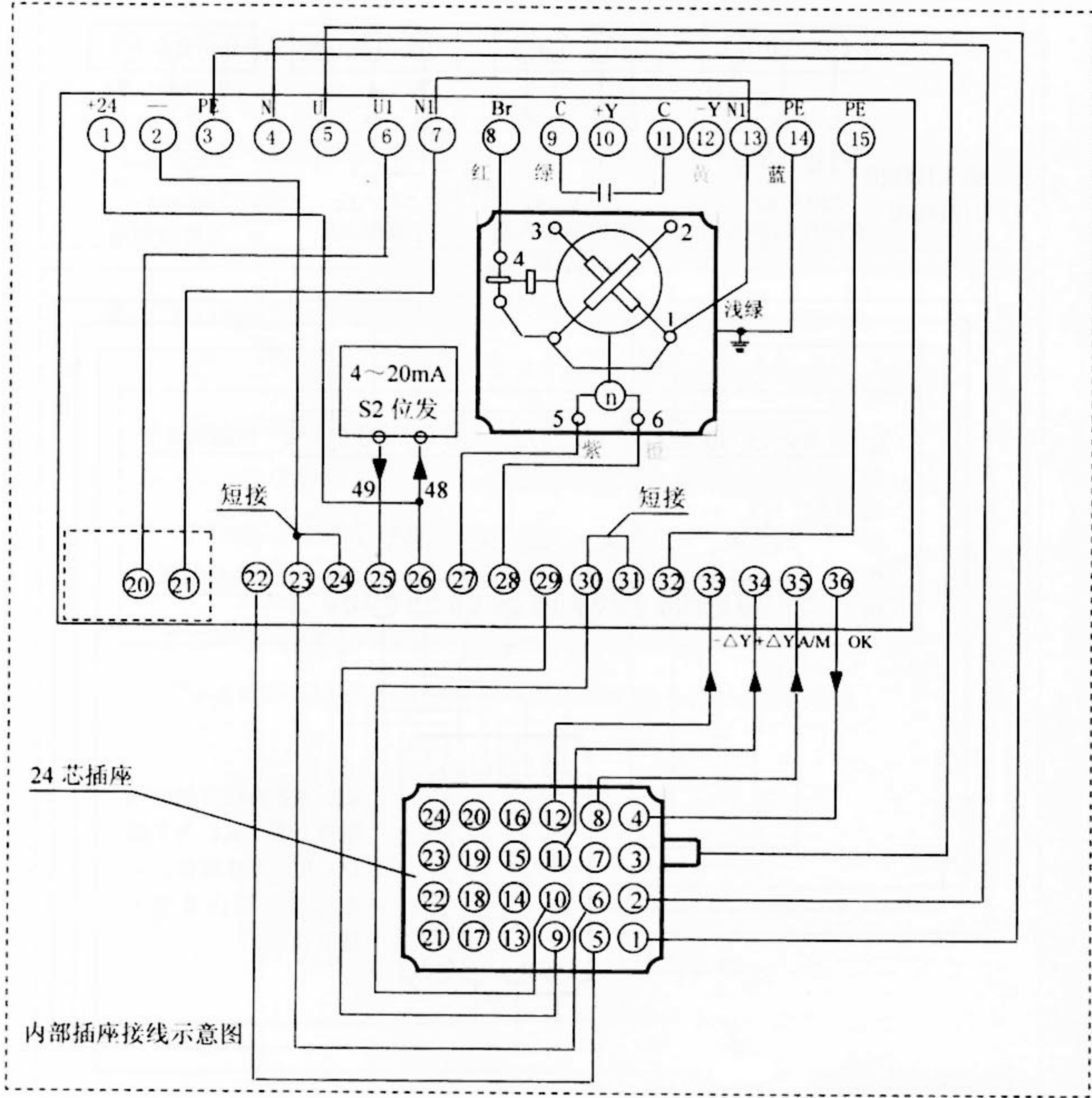
RHD 调节型一体化 (T) 电动执行机构接线图
