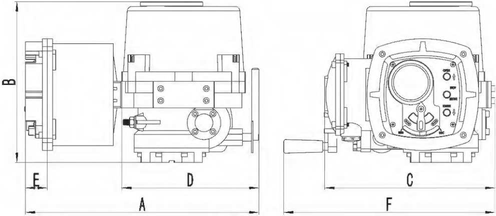
直连式外形尺寸图
